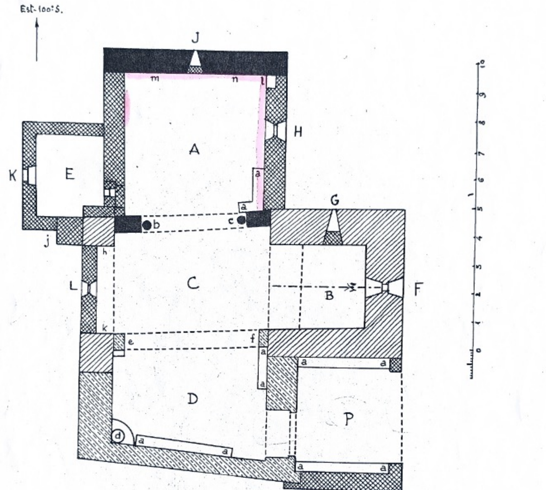
Fig. A: Plan schématique, à DIX Millimètres pour UN Mètre.
